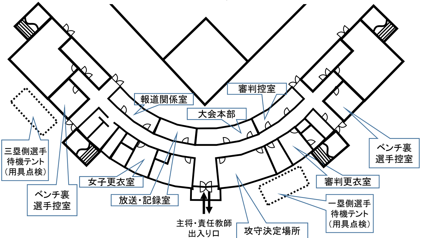
あやべ球場本部棟平面図
